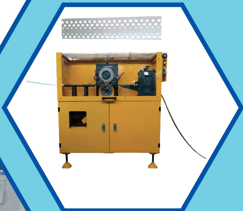
MÁY ĐỘT LỖ Rotary Punching Machine
