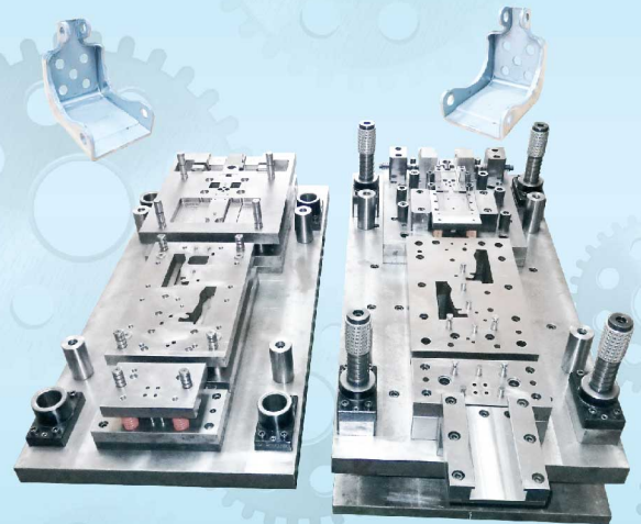
KHUÔN DẬP LIÊN HOÀN Progressive Stamping Mold
