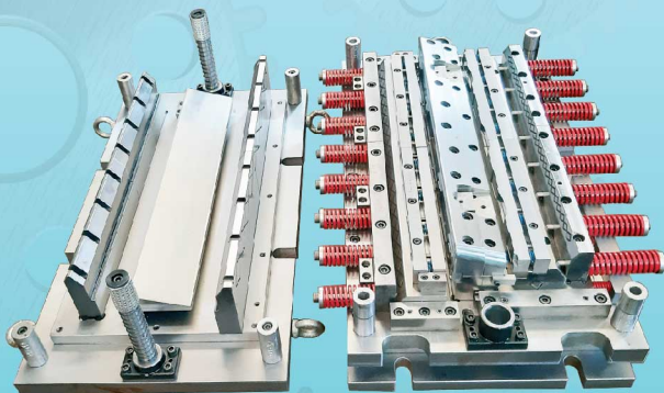
KHUÔN DẬP VUỐT Forming Mold
