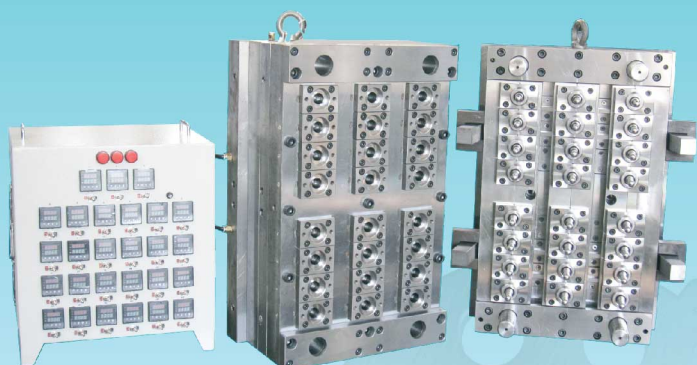
KHUÔN ÉP PHÔI PET - 24 CAV 24 CAV - PET Preform Mold
