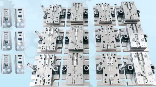
KHUÔN DẬP LIÊN HOÀN Progressive Stamping Mold
