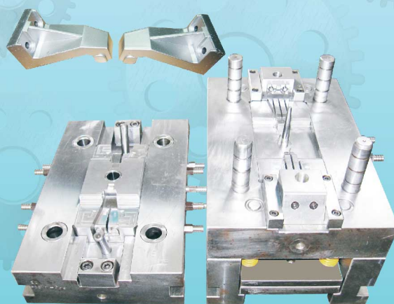
KHUÔN ĐÚC ÁP LỰC Die - Casting Mold
